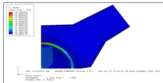
Gambar 4. Kontur von Mises stress CoCr-on-ST.
