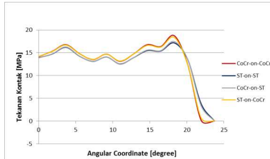
Gambar 10. Distribusi tekanan kontak pada metal-on-metal .
