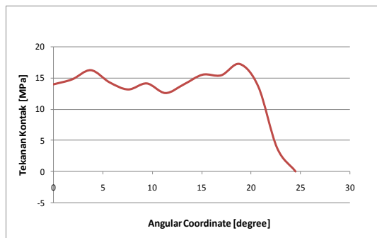
Gambar 9. Distribusi tekanan kontak ST-on-ST
