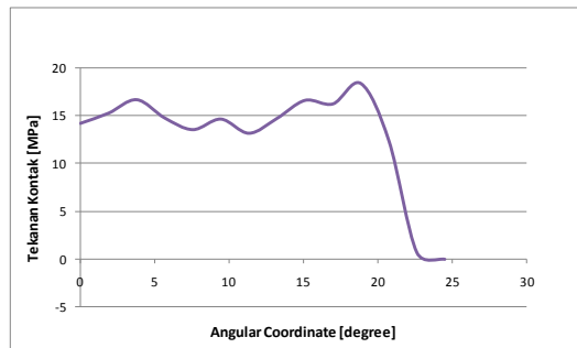
Gambar 7. Distribusi tekanan kontak ST-on-CoCr
