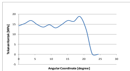
Gambar 3. Distribusi tekanan kontak CoCr-on-CoCr
