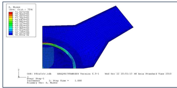
Gambar 6. Kontur von Mises stress ST-on-CoCr.
