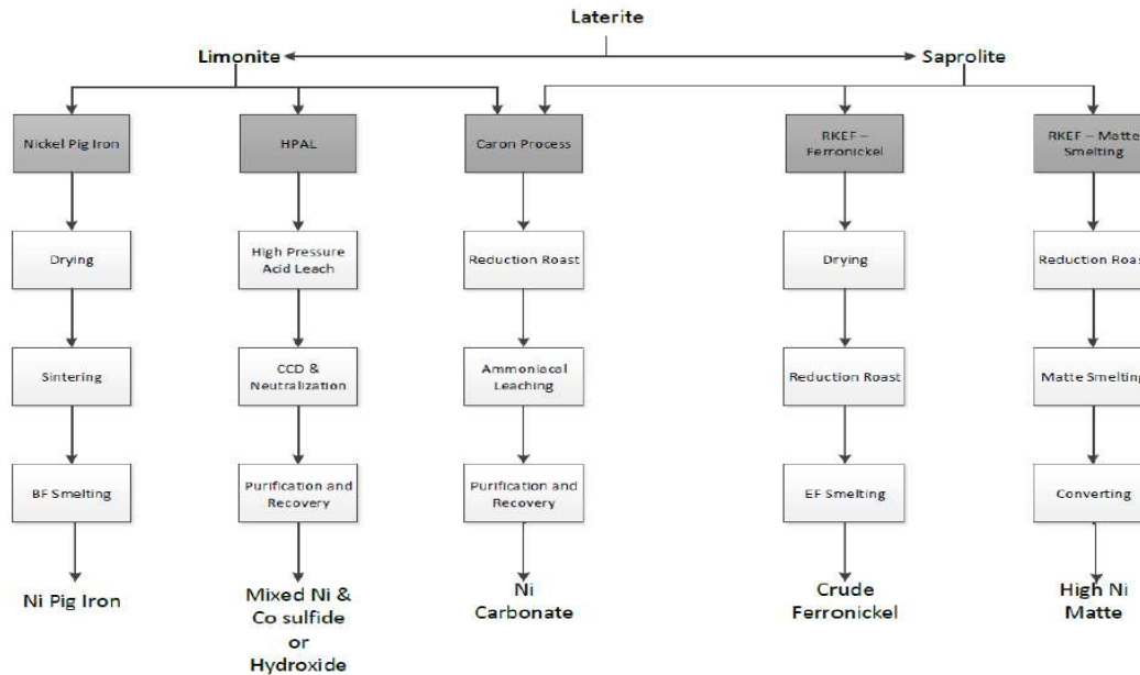
Gambar 3. Diagram Alir Proses Pengolahan Laterit. 9)
