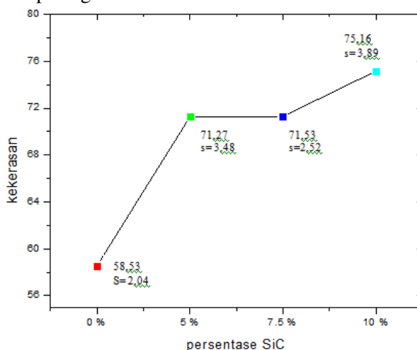
Gambar 5. Hubungan antara kekerasan dengan persentase SiC
