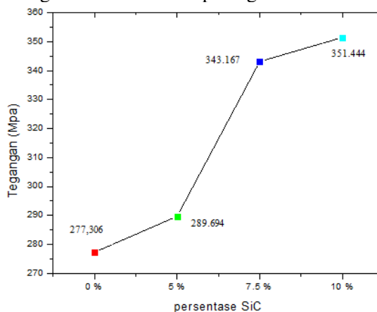
Gambar 6. Hubungan antara tegangan dengan persentase SiC
