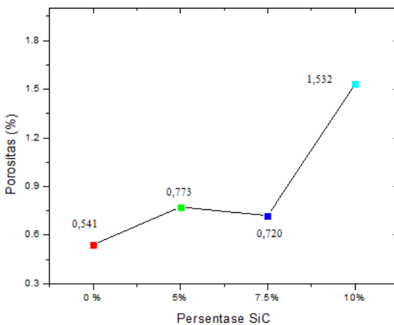
Gambar 4. Grafik hubungan antara porositas terhadap persentase SiC
