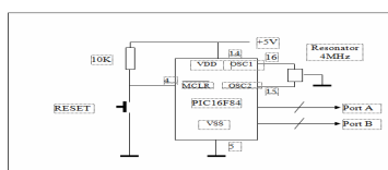
Gambar 7 Sistem mikrokontroler PIC16F84
