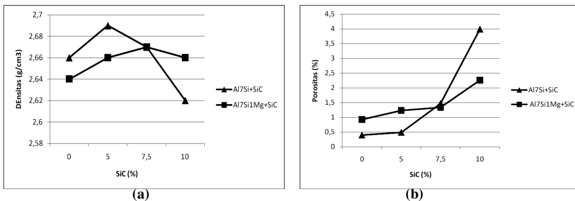
Gambar 2. Grafik (a) densitas, (b) tingkat porositas komposit
