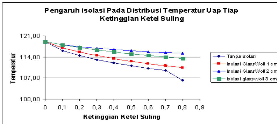
Gambar 4. pengaruh isolasi glashwoll terhadap temperatur uap
