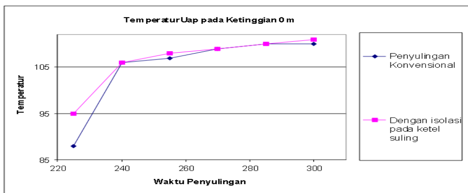
Gambar 5. Temperatur uap pada ketinggian 0 m dari permukaan air untuk dua variasi penyulingan
