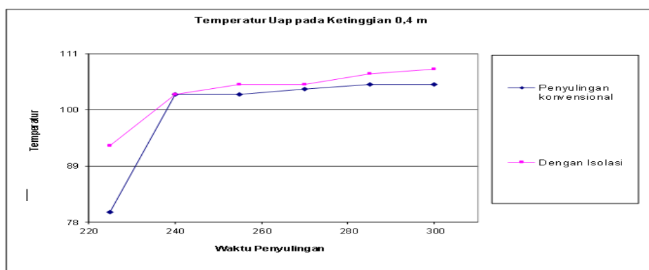
Gambar 6. Temperatur uap pada ketinggian 0,4 m dari permukaan air untuk tiga variasi penyulingan
