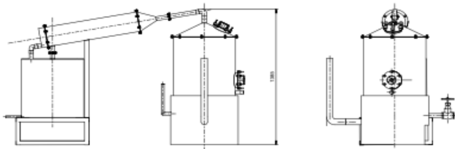
Gambar 2 Penyulingan minyak atsiri
