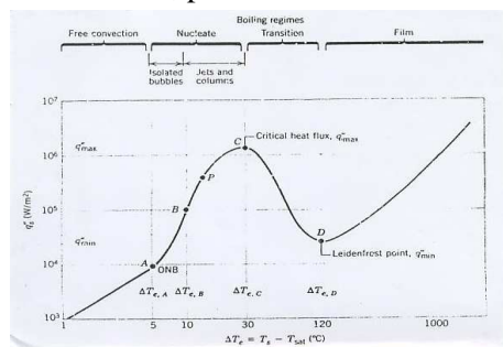
Gambar 1. Kurva tipe pendidihan untuk air pada tekanan atmosfer
