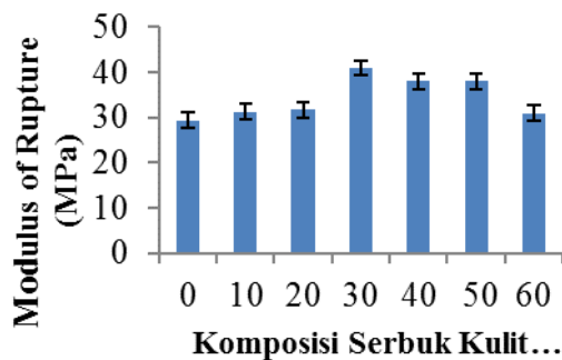
Gambar 2 Pengaruh Variasi Komposisi Pengisi Serbuk Kulit Kerang Terhadap Keteguhan Patah ( Modulus of Rupture ) Papan Partikel.
