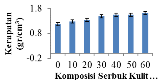
Gambar 1 Pengaruh Variasi Komposisi Pengisi Serbuk Kulit Kerang Terhadap Kerapatan Papan Partikel
