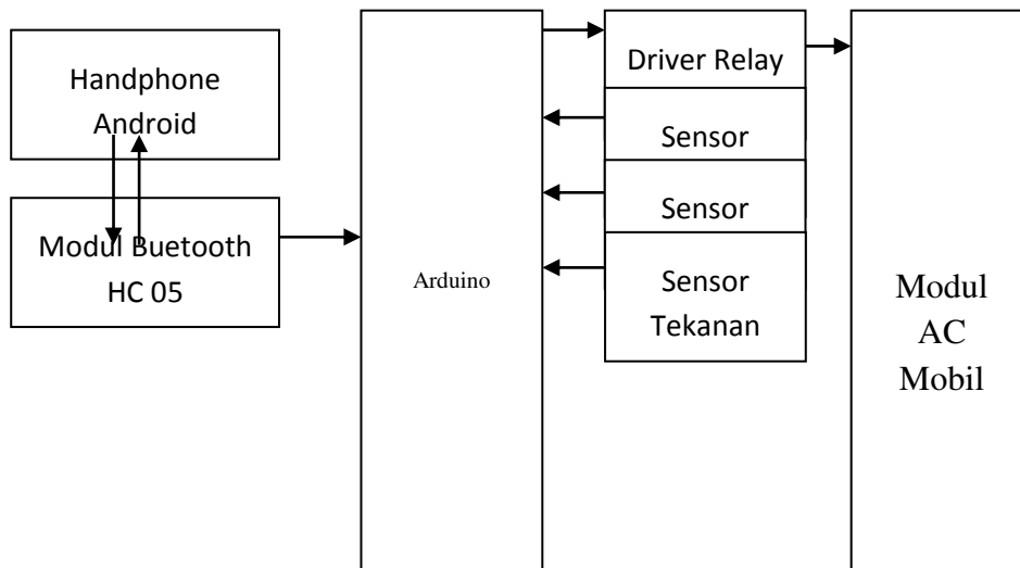
Gambar 2. Skema perancangan alat
