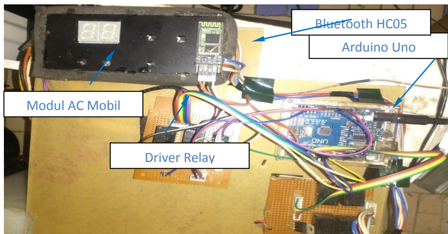
Gambar 3. Susunan perangkat sistem kontrol
