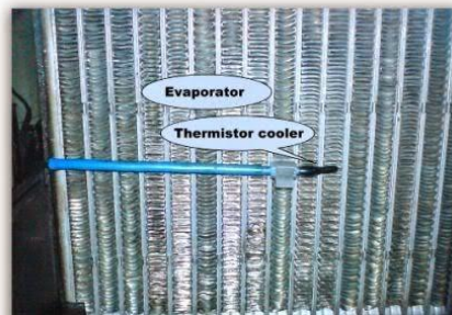
Gambar 5. Perangkat sensor suhu
