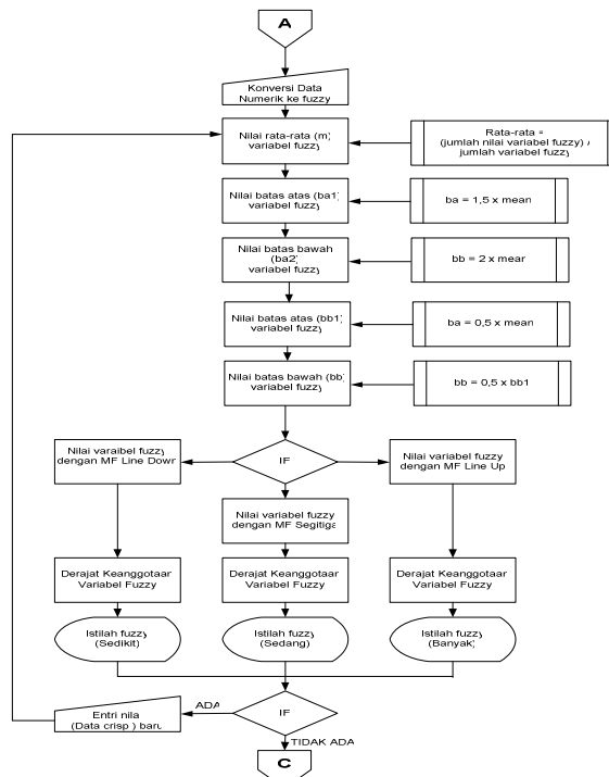
Gambar 3.2 Tahapan Konversi Nilai Crisp ke Fuzzy
