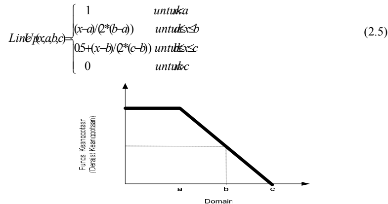
Gambar 2.4 Grafik Fungsi Keanggotaan Line Down (Bezdek, B & C. James, 1993)
