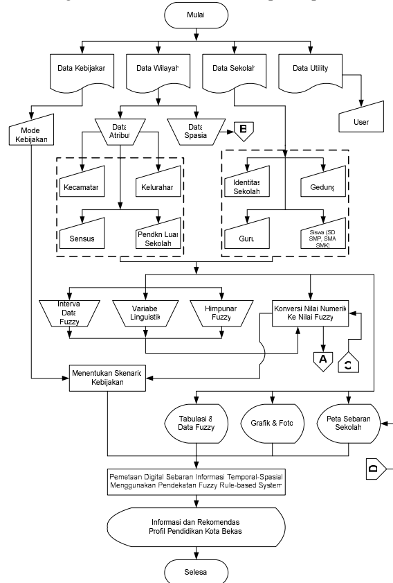
Gambar 3.1 Tahapan Implementasi FRBS
