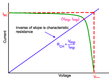
Gambar 2.4 Karakteristik resistansi [2]
