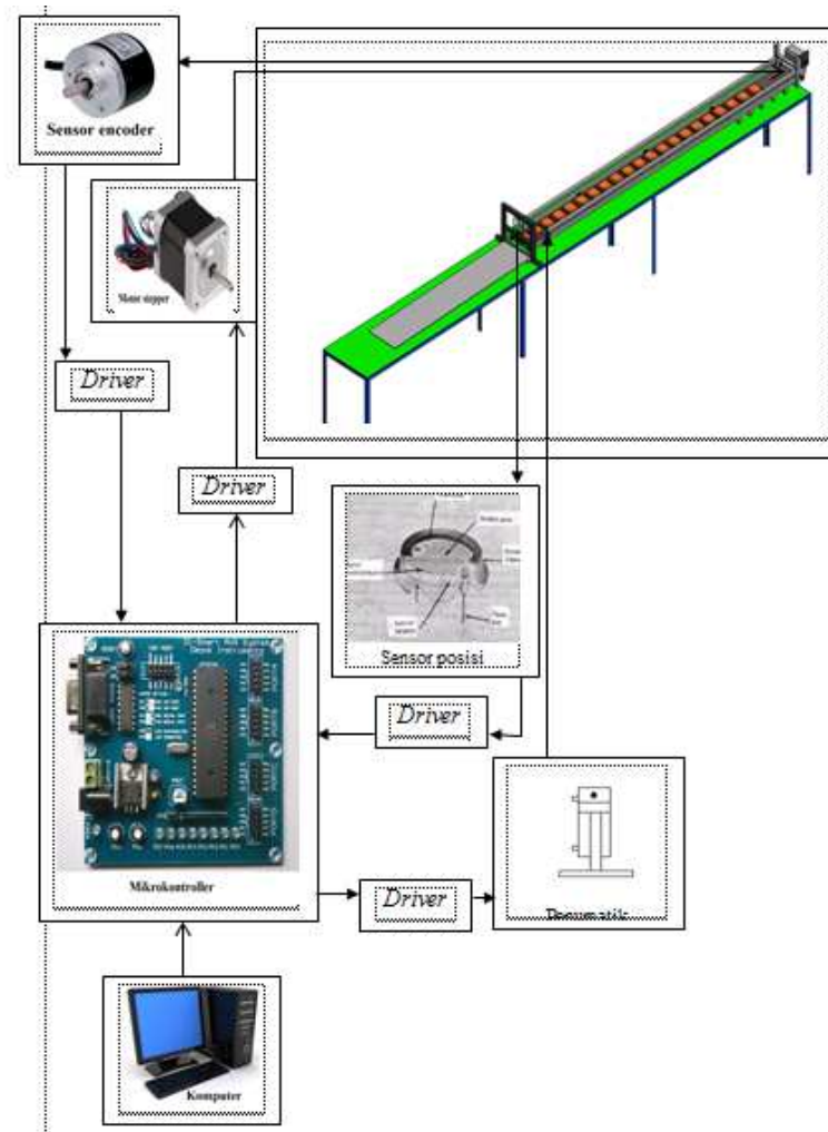
Gambar 3. Perancangan Hardwar
