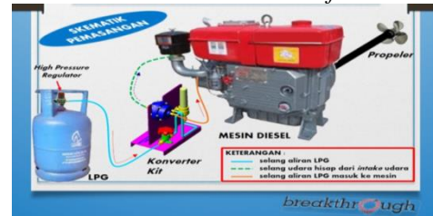
Gambar 6. Skema kerja sistem dual-fuel .
