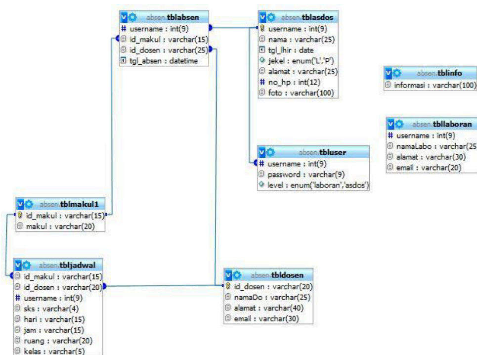
Gambar 4: Relasi tabel
