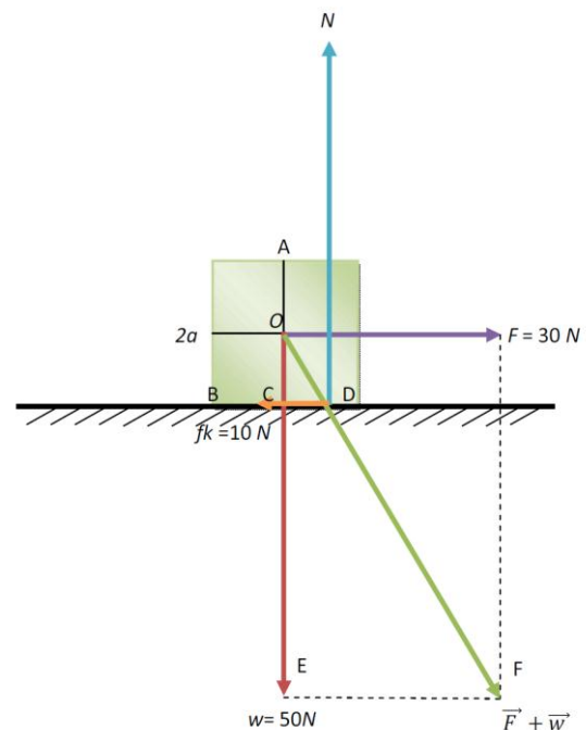
Gambar 2. Diagram gaya pada kubus dengan sisi 2a yang ditarik dengan gaya F
