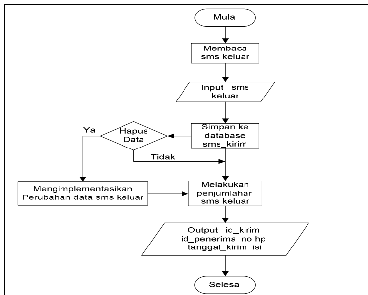
Gambar 3.4 PSPEC Lihat Data SMS Keluar
