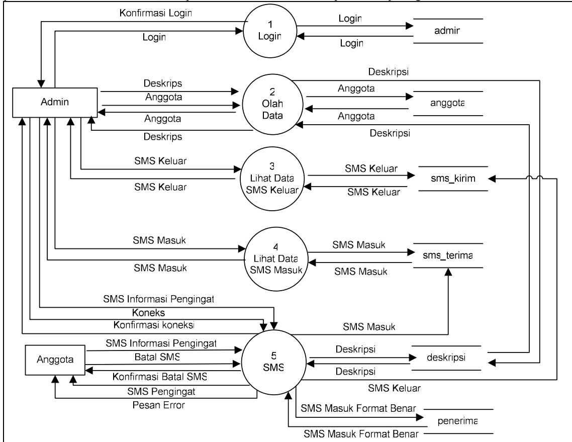
Gambar 3.3 DFD Level 1 Aplikasi SMS Peningkat Ibu Hamil
