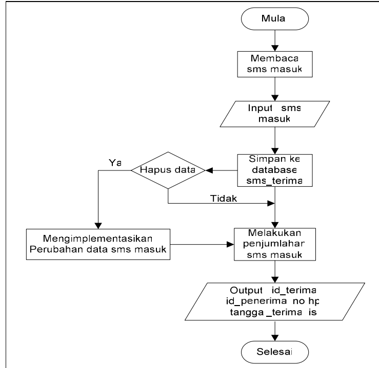
Gambar 3.5 PSPEC Lihat Data SMS Masuk
