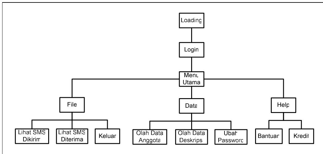
Gambar 3.8 Rancangan AntarMuka
