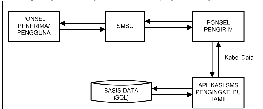
Gambar 3.1 Arsitektur Sistem
