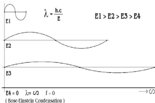
Gambar 1. Hubungan Panjang Gelombang, Frekuensi dan Energi
