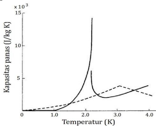
Gambar 2. Kapasitas Panas Helium Cair
