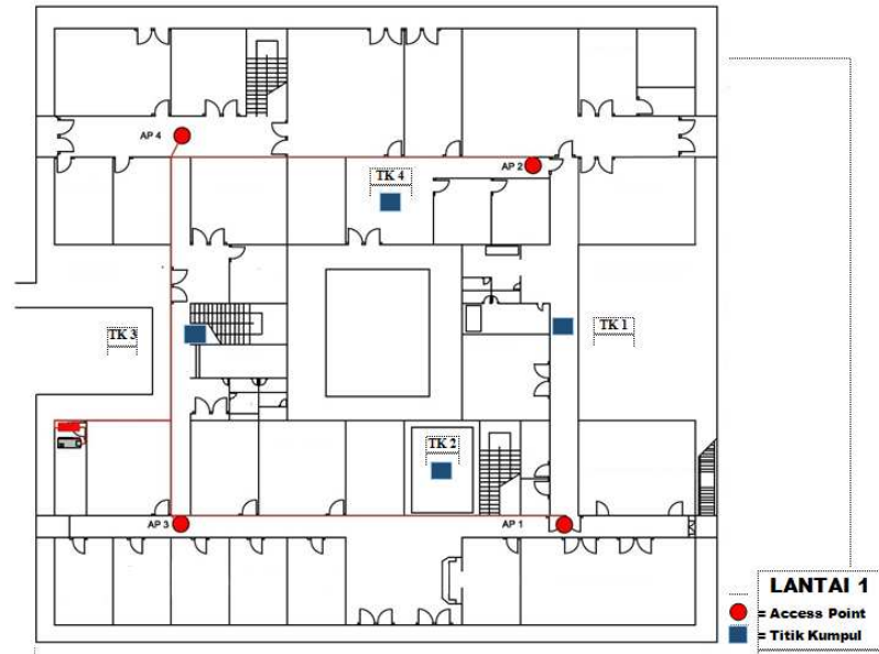
Gambar 2. Denah lokasi lantai 1
