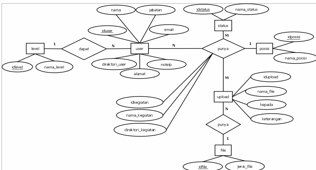
Gambar 5. Perancangan ERD Aplikasi Manajemen File
