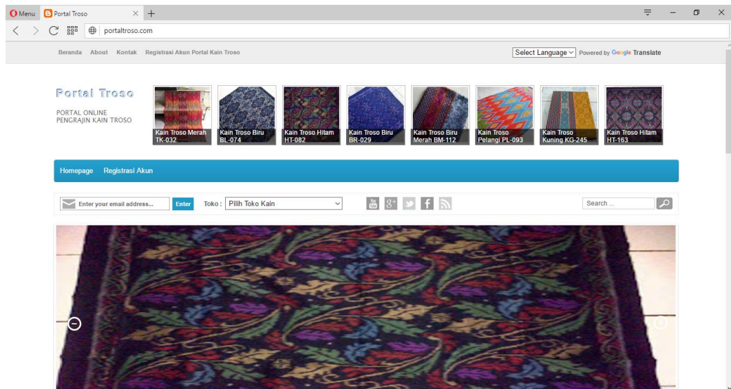
Gambar 2 Tampilan Awal
