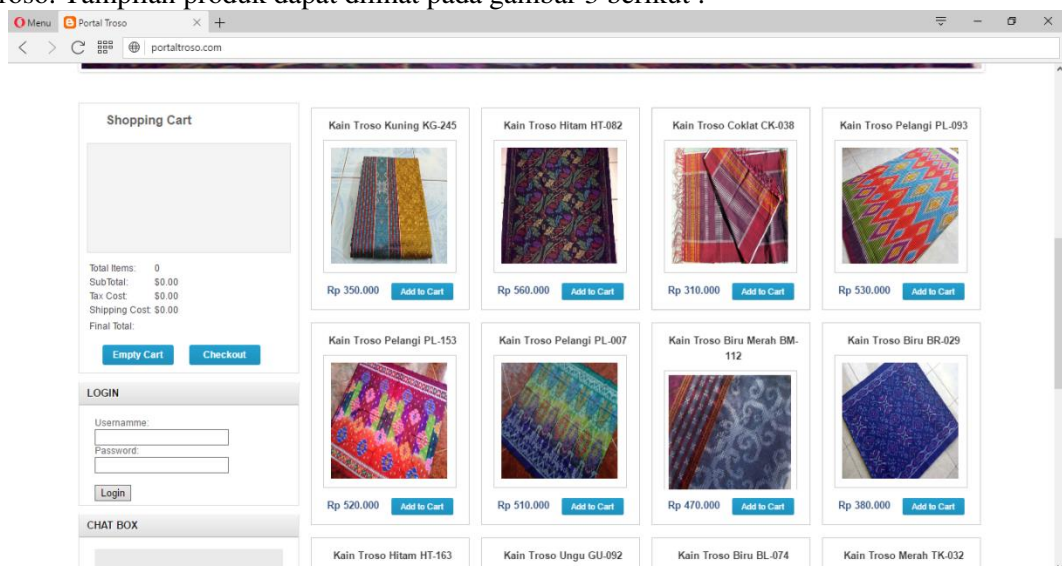
Gambar 3 Tampilan Produk
