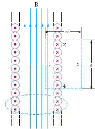
Gambar 1. Arah arus kumparan dan arah garis gaya magnet
