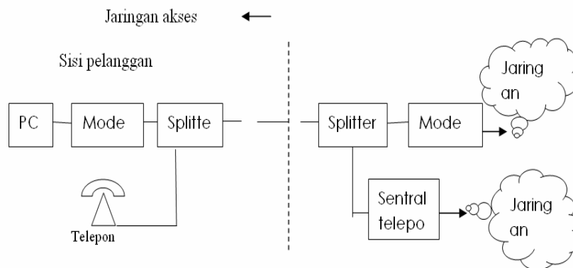
Gambar 6. Diagram instalasi implementasi ADSL pada jaringan akses telepon tetap. Sumber: Allurayeff (2012)e
