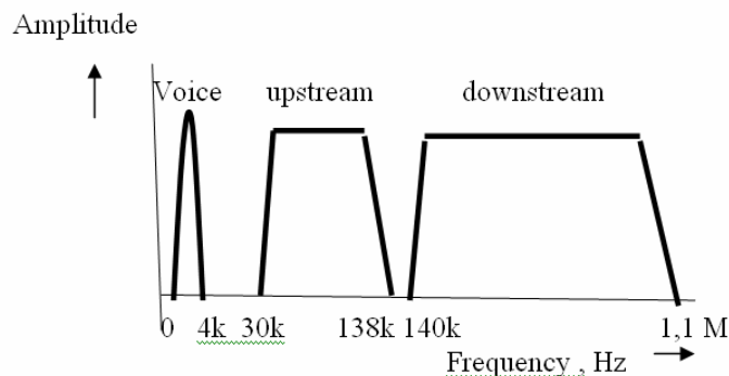
Gambar 2. Pembagian Kanal Lebar Pita Frekuensi ADSL Sumber :Brito (2012)
