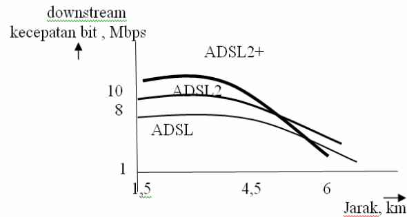
Gambar 5. Hubungan bit rate dengan jarak untuk ADSL, ADSL2 dan ADSL2+. Sumber : Hens (2008)
