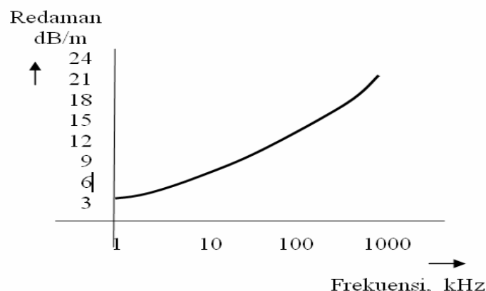
Gambar 1. Hubungan Redaman terhadap Frekuensi untuk Kawat Tembaga Diameter 0,016 inci (tipe 24 AWG)
