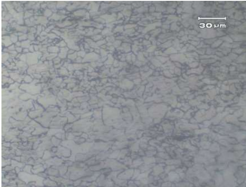
Gambar 7. Struktur mikro baja laterit hasil pengerolan panas dengan reduksi 30-35%. Pembesaran 500x. Etsa Nital 2%
