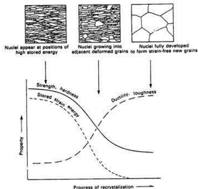
Gambar 1. Skema proses rekristalisasi (Alexander & Davies, 1985).
