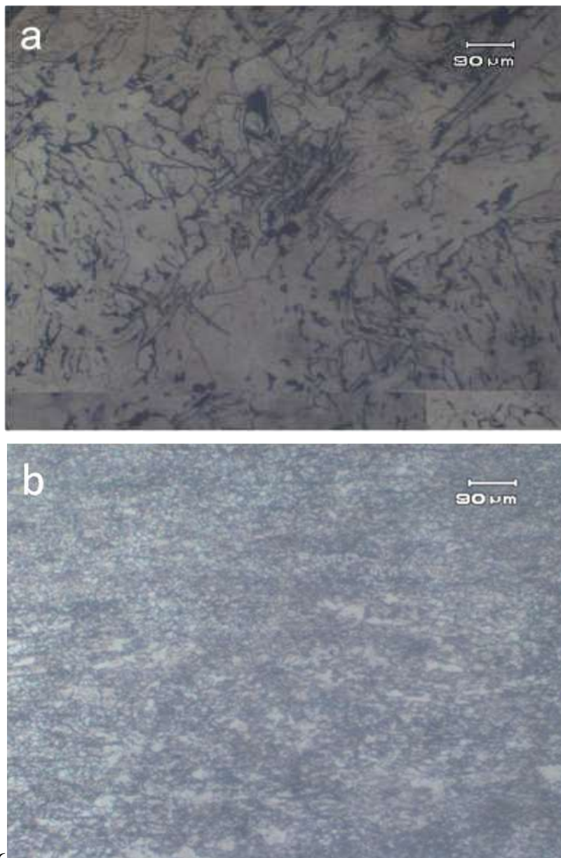
Gambar 6. Struktur mikro baja a) kondisi as-cast dan b) hasil pengerolan panas reduksi 30-35%. Pembesaran 100x. Etsa Nital 2%
