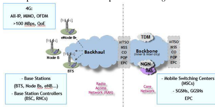
Gambar 2. Jaringan backhaul-backbone pada komunikasi seluler
