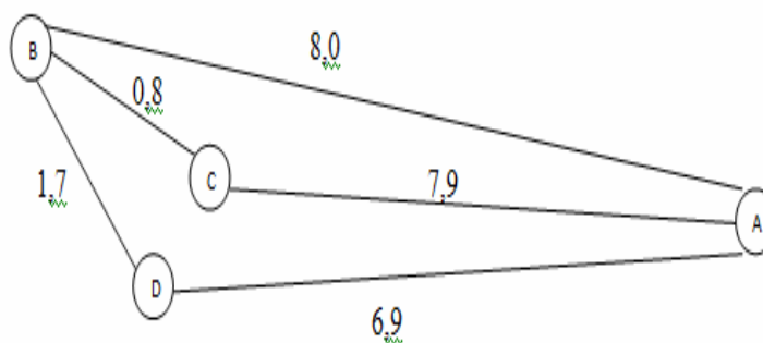
Gambar 6. Graf Rute
