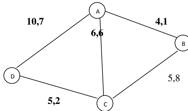
Gambar 3. Graf Rute
