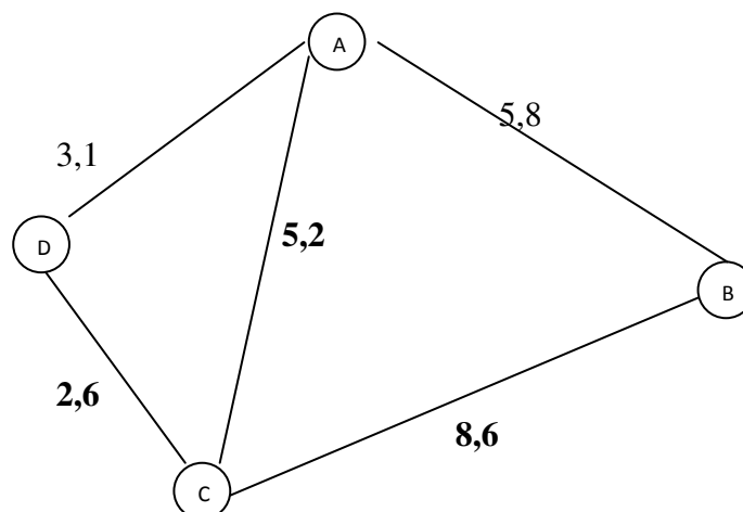
Gambar 4. Graf Rute
