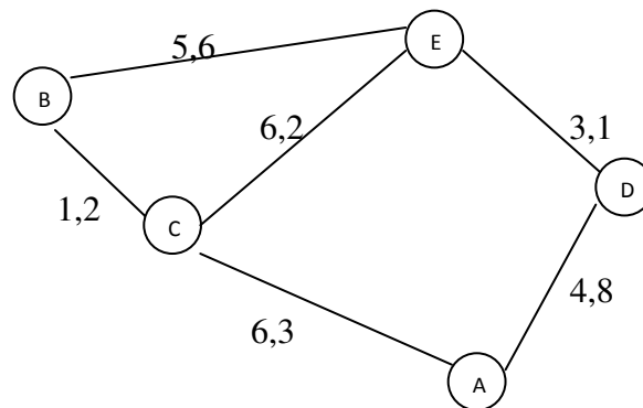
Gambar 5. Graf Rute
