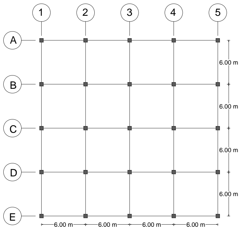
Gambar 2. Denah Bangunan
