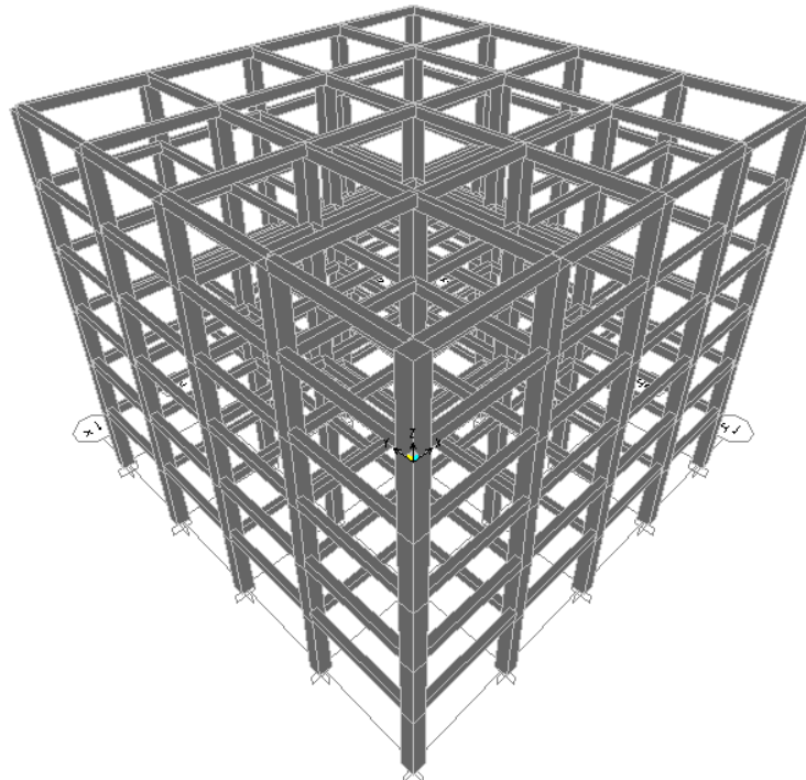
Gambar 3. Struktur 3 Dimensi
