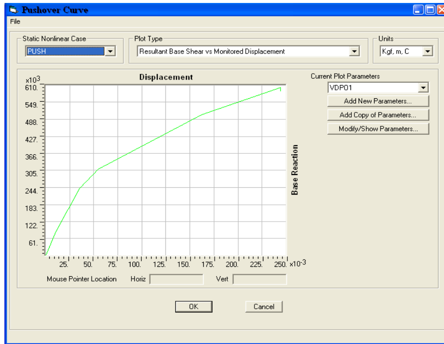
Gambar 4. Kurva Pusover
