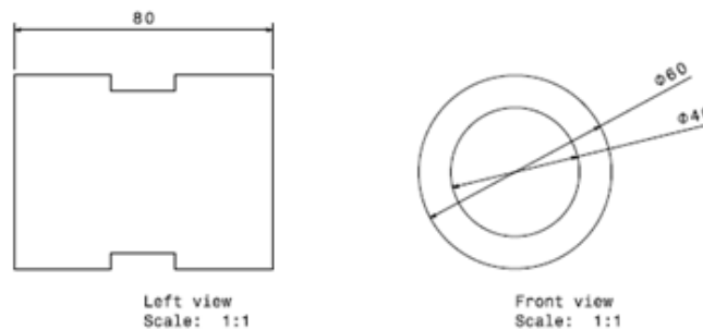
Gambar 4.5. Sambungan Piston
