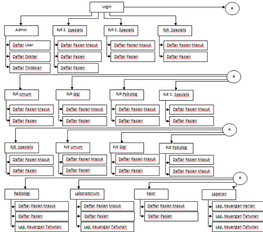
Gambar 2. Struktur Navigasi
