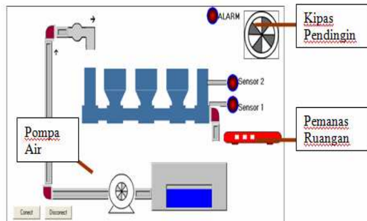
Gambar 2 Rancangan Skema Web Browser
