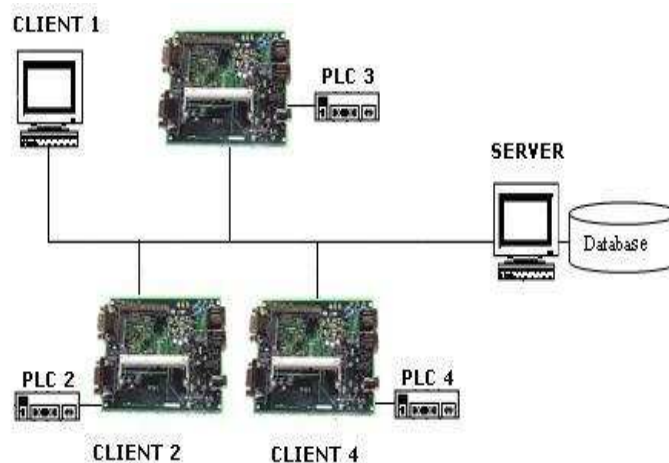
Gambar 6. Kerja Server
