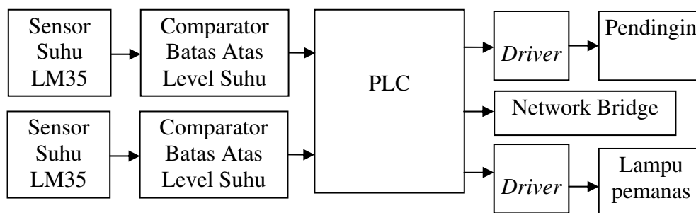
Gambar 3. Blok Diagram Perangkat Keras
