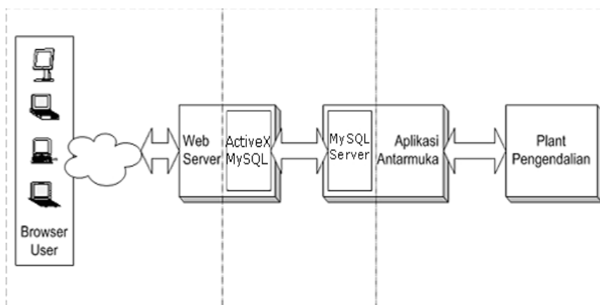
Gambar 1. Rancangan Skema Web Server
