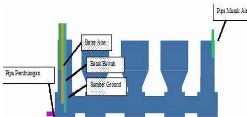
Gambar 4. Perancangan Sensor Ketinggian Level Air
