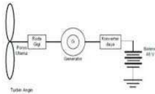
Gambar 1 Skema Konversi Energi Angin Sumber: lugiromadoni.blogspot.com
