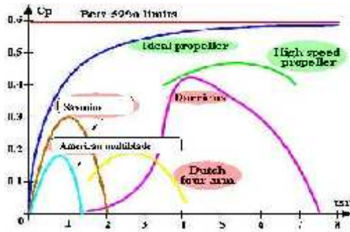
Gambar 5: diagram hub Cp dan TSR
