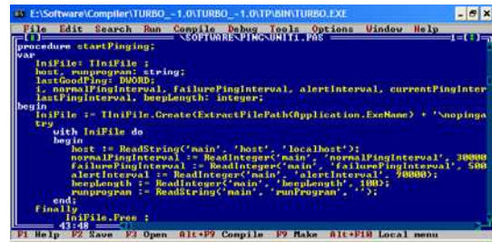
Gambar 2. Tampilan Source Code Bahasa Pemrograman Pascal Saat Start Ping
