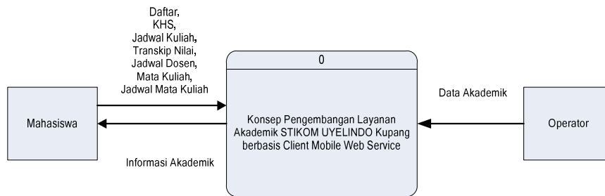
Gambar 2. Digram Konteks
