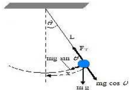
Gambar.1 Bandul Matematis
