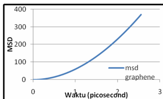
Gambar 12. Grafik MSD simulasi Graphene
