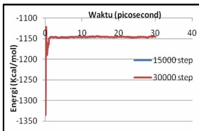
Gambar 6. Grafik trajektori energi simulasi Argon 256 atom
