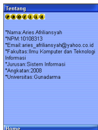
Gambar 5. Tampilan Tentang
