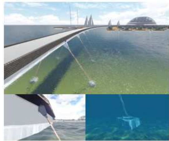
Gambar 4. Sistem anker yang diterapkan pada J3F
