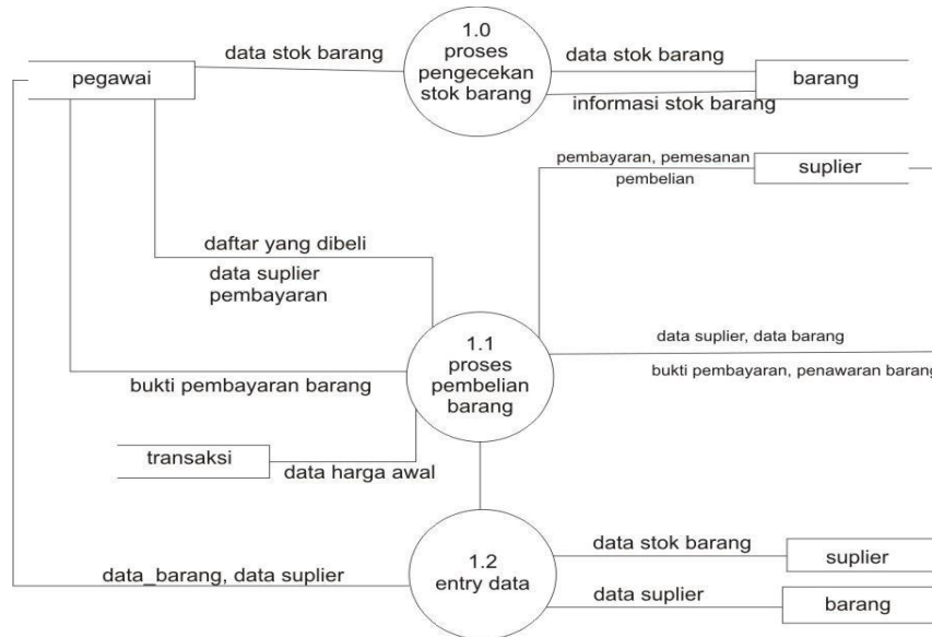
Gambar 3 : DFD Level 0
