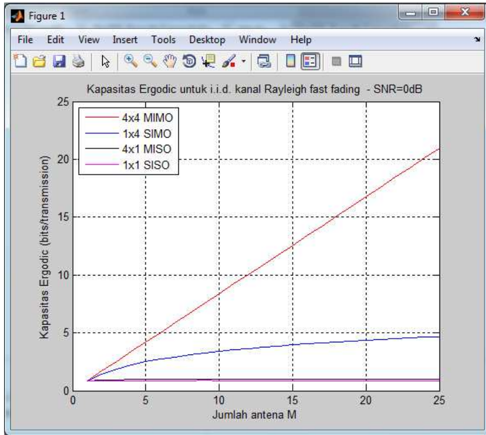
Gambar 4 Pengaruh jumlah antena
