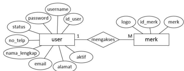
Gambar 3. Relasi entitas user dan merk
