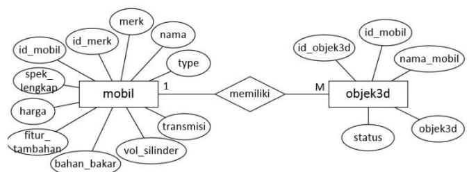
Gambar 5. Relasi entitas mobil dan objek3d
