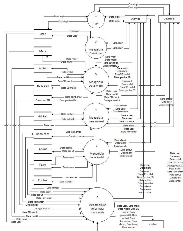
Gambar 2. DFD level 1
