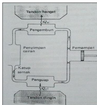
Gambar 2. Instalasi Pendingin Dasar (Sumber: Zemasky & Ditman, 1986)
