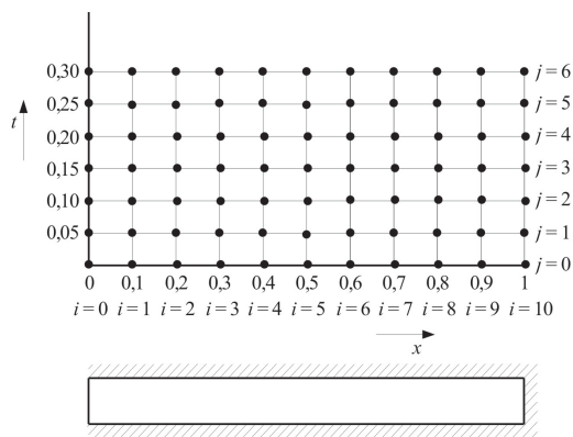
GAMBAR 5: Grid untuk kasus gambar 4
