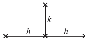
GAMBAR 2: Keempat titik pada pers.(7)
