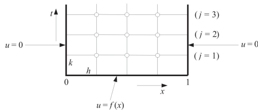
GAMBAR 1: Grid dan titik-titik mesh untuk pers.(7)
