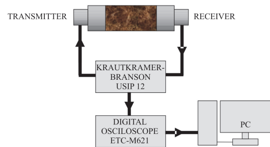
GAMBAR 3: Diagram blok pengukuran
