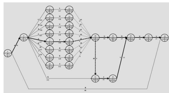
Gambar 6. Jaringan Kerja dan Lintasan Kritis dengan Percepatan Waktu Penyelesaian kegiatan X
