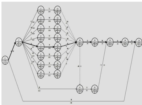
Gambar 1. Jaringan Kerja dengan Waktu Normal
