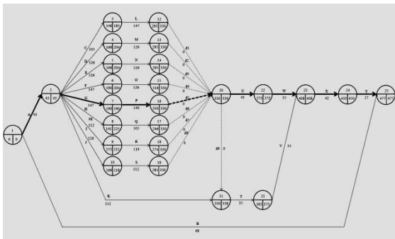
Gambar 4. Jaringan Kerja dan Lintasan Kritis dengan Percepatan Waktu Penyelesaian kegiatan A
