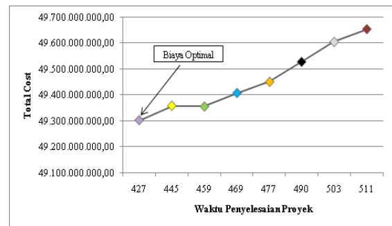
Gambar 9. Grafik Perubahan Total Cost terhadap Waktu Penyelesaian Proyek
