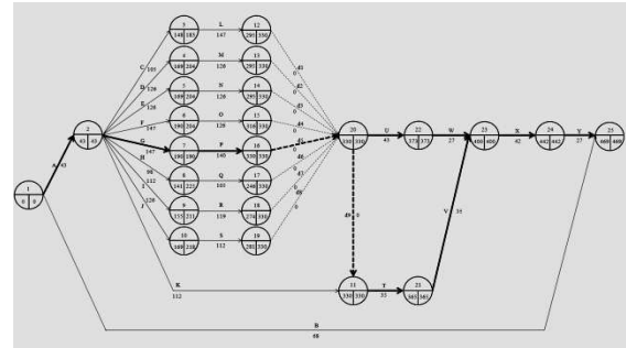
Gambar 5. Jaringan Kerja dan Lintasan Kritis dengan Percepatan Waktu Penyelesaian kegiatan W
