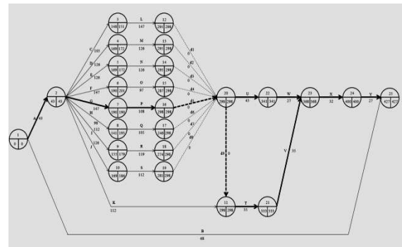
Gambar 8. Jaringan Kerja dan Lintasan Kritis dengan Percepatan Waktu Penyelesaian kegiatan O
