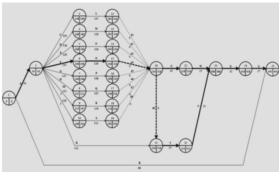
Gambar 7. Jaringan Kerja dan Lintasan Kritis dengan Percepatan Waktu Penyelesaian kegiatan P
