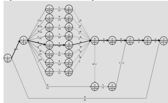
Gambar 2. Jaringan Kerja dan Lintasan Kritis dengan Percepatan Waktu Penyelesaian kegiatan Y
