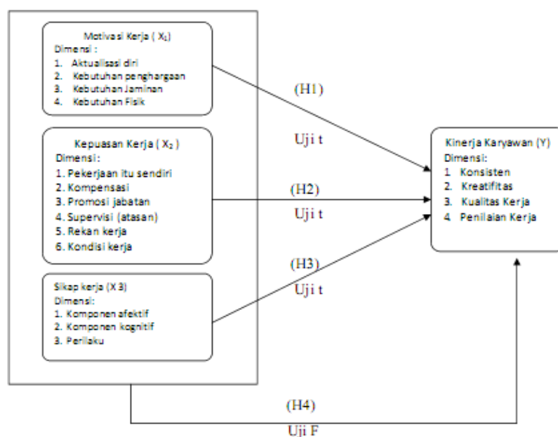
Gambar 1 Kerangka Pemikiran
