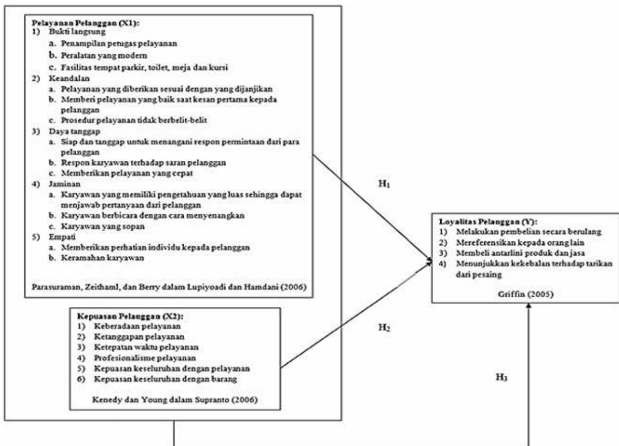
Gambar 1 Kerangka Pemikiran
