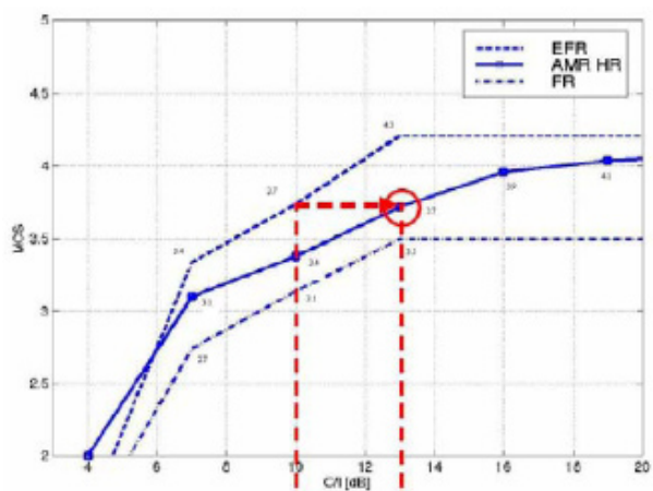
Gambar 7 Perbandingan Kanal EFR dan AMR Halfrate
