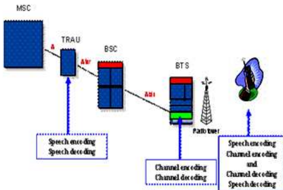
Gambar 1 Penerapan AMR pada GSM
