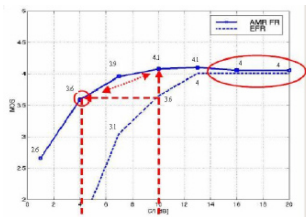
Gambar 6 Perbandingan Kanal EFR dan AMR Fullrate
