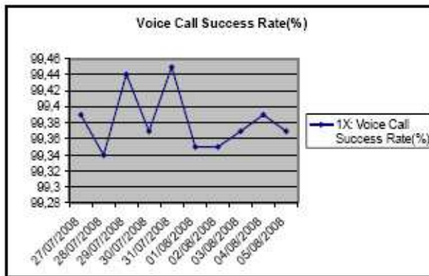
Gambar 8 Statistik Call Success Rate pada BTS AMR
