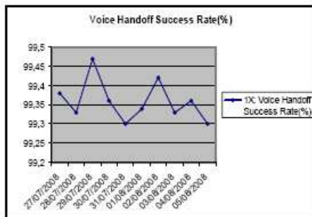
Gambar 10 Statistik Handover Success Rate pada BTS AMR
