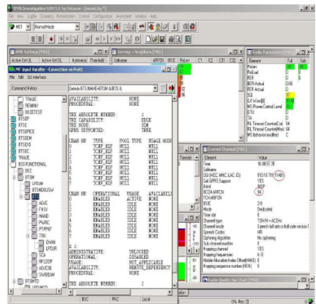
Gambar 4 Data TEMS SQI Call Non Amr Halfrate
