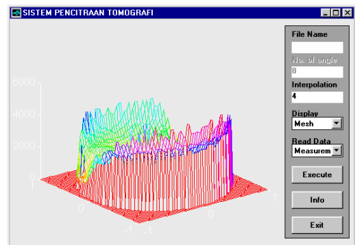
Gambar 10 Hasil Rekonstruksi Interpolasi dengan Jumlah Sensor Identik 128 Transduser dengan 3 Medium Gas, Lumpur, dan Pasir
