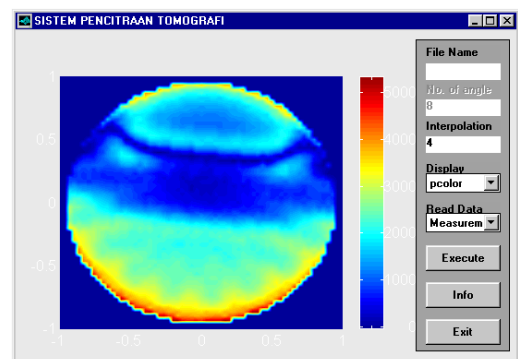
Gambar 11 Hasil Rekonstruksi Interpolasi dengan Jumlah Sensor Identik 128 Transduser dengan 3 Medium Gas, Air, dan Pasir
