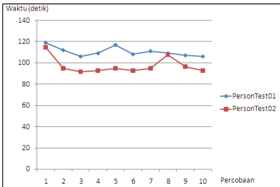
Grafik 2 Grafik perbandingan antara tabel PersonTest01 dan PersonTest02 sesudah diberi index
