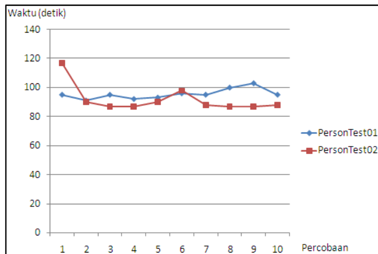
Grafik 1 Grafik perbandingan antara tabel PersonTest01 dan PersonTest02 sebelum diberi index
