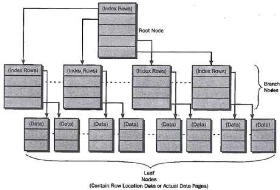
Gambar 1 Struktur Index
