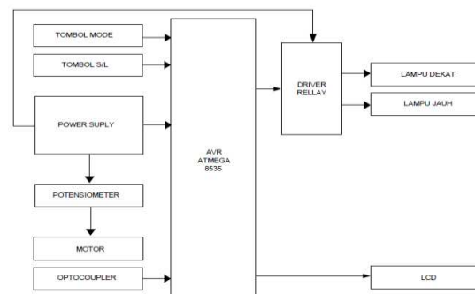
Gambar 3.1. Blok diagram kotak Sistem pengendali lampu jarak jauh dan dekat pada kendaraan secara otomatis
