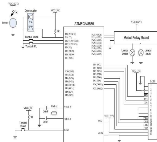
Gambar 3.2 rangkaian keseluruhan
