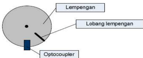
Gambar 2.2. Sensor kecepatan
