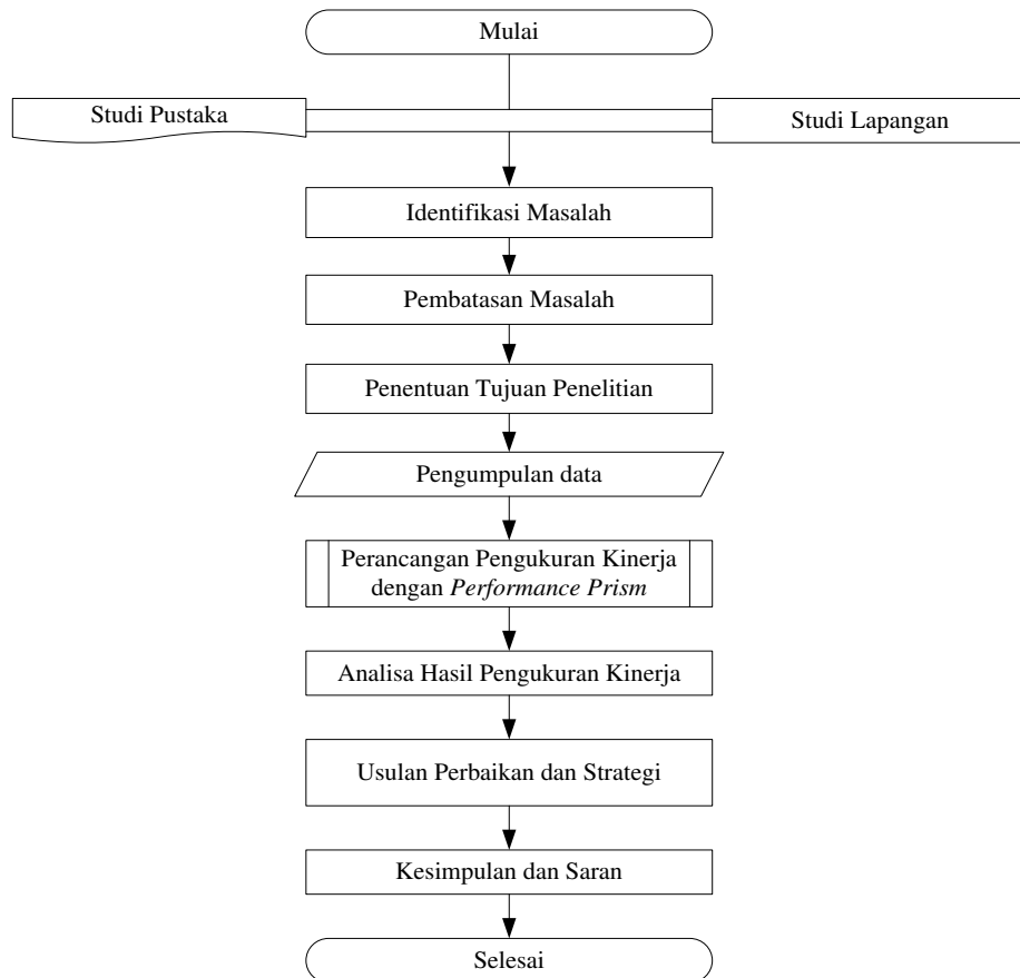
Gambar 1. Metodologi Penelitian
