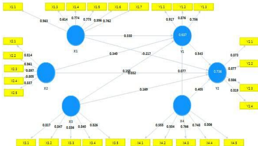
Gambar 2. Diagram Jalur Persamaan Struktural Efektivitas SIKD Pemkab Jembrana
